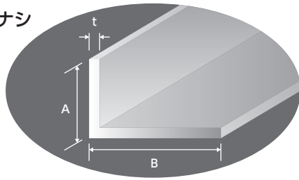
■寸法(Rナシ)
