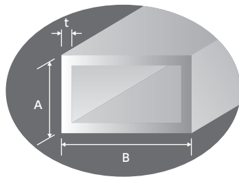
■平角管寸法 長さ=5000mm
