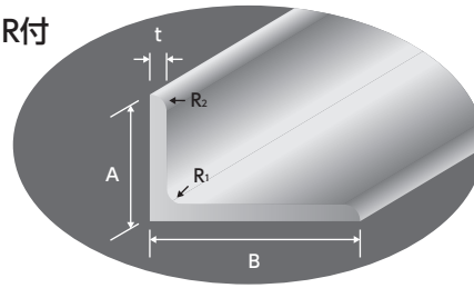
■寸法(R付)
